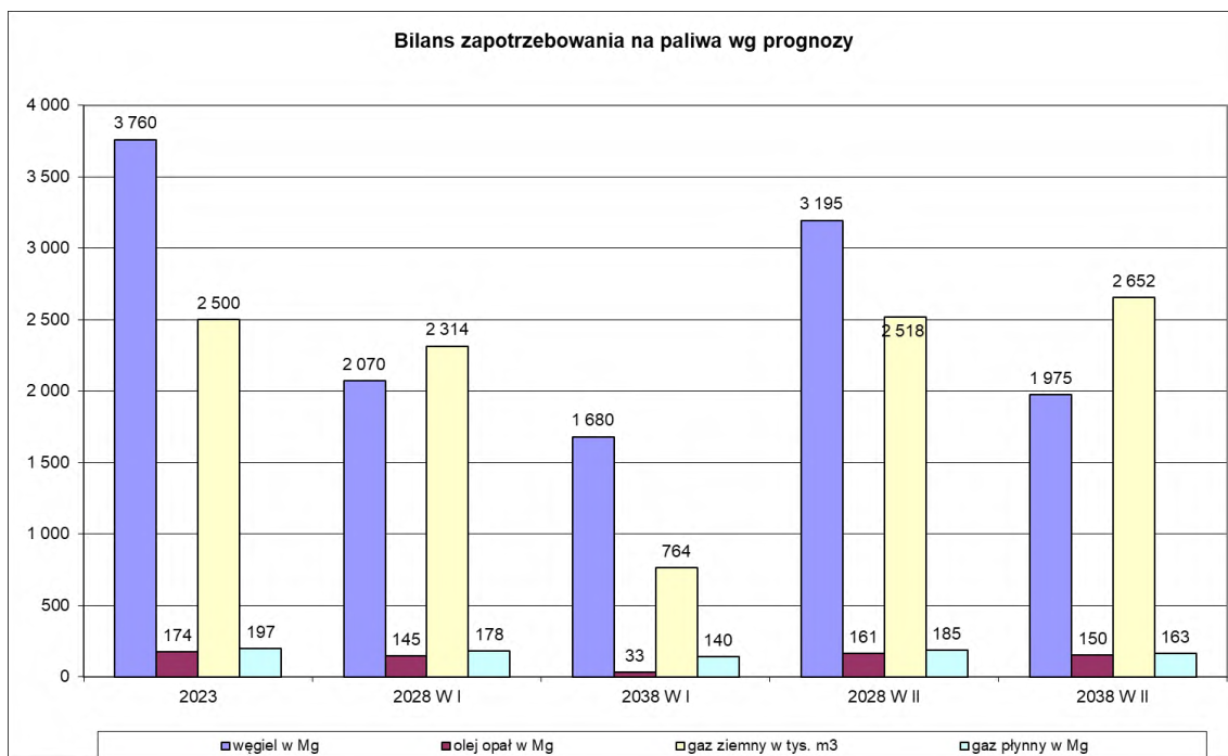
Wykres 2. Prognoza zużycia paliw w latach 2028 – 2038
