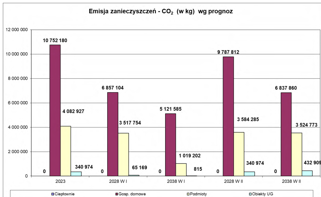
Wykres 8. Emisja zanieczyszczeń - CO 2 (w kg) w latach 2023 - 2038
